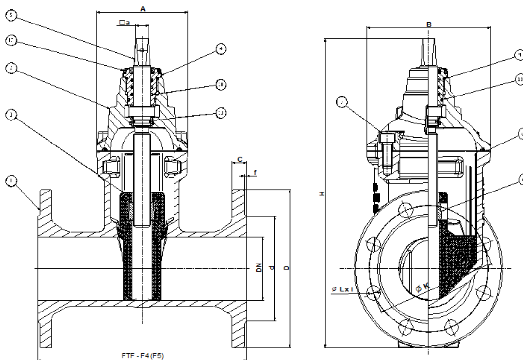
Rys. 1 – Budowa zasuw zaporowej
